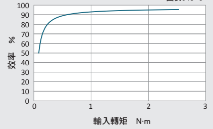
【減速比=20、25】
